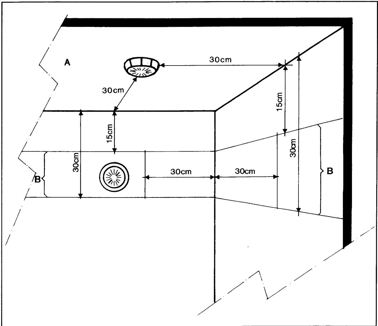
➔ Figure 2: A = zone d'implantation des détecteurs au plafond, le plus au centre possible, mais à une distance minimale de 30 cm de tous les coins et bords du plafond; B = zone d'implantation admise sur les murs à 15 cm minimum et 30 cm maximum du plafond et à 30 cm minimum d'un coin.
