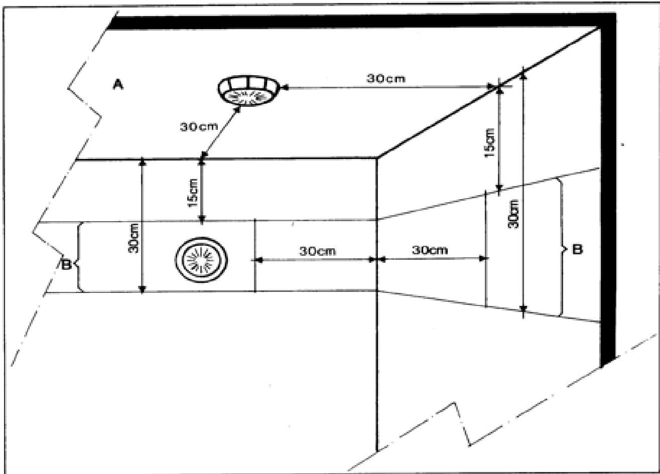
➔ Figuur 2: A = zone waar een detector aan het plafond kan worden bevestigd, zo dicht mogelijk bij het midden maar op minimum 30 cm van alle hoeken en randen van het plafond; B = zone waar een rookdetector aan de wand mag worden bevestigd, op minimum 15 cm en maximum 30 cm van het plafond en op minimum 30 cm van een hoek.
